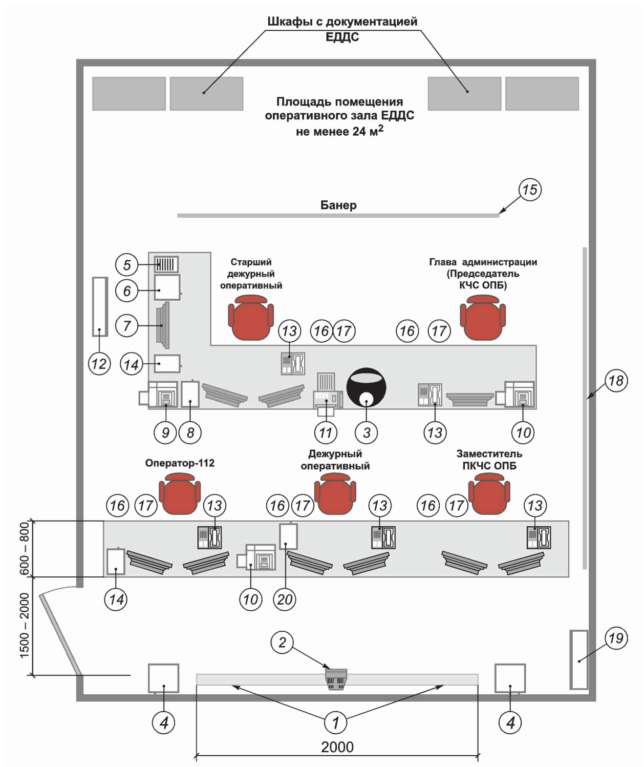
Рисунок А.1 - Примерная схема размещения рабочих мест и оборудования ЕДДС
